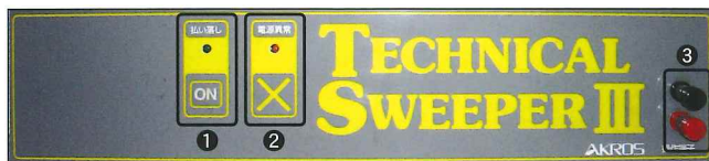
①チリ落とし作動スイッチと表示 ②電源異常表示 ③操作線接続端子
